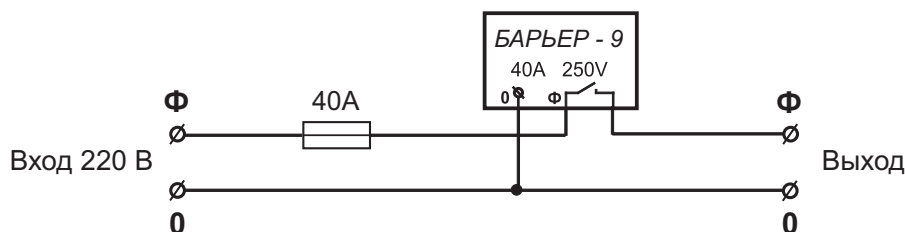
Рис.1 Схема подключения прибора. В качестве предохранителя может быть токвый автомат. Предохранитель или токвый автомат обязательные элементы схемы подключения прибора.
